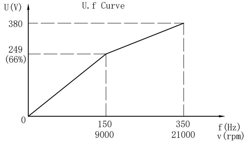
频压曲线
