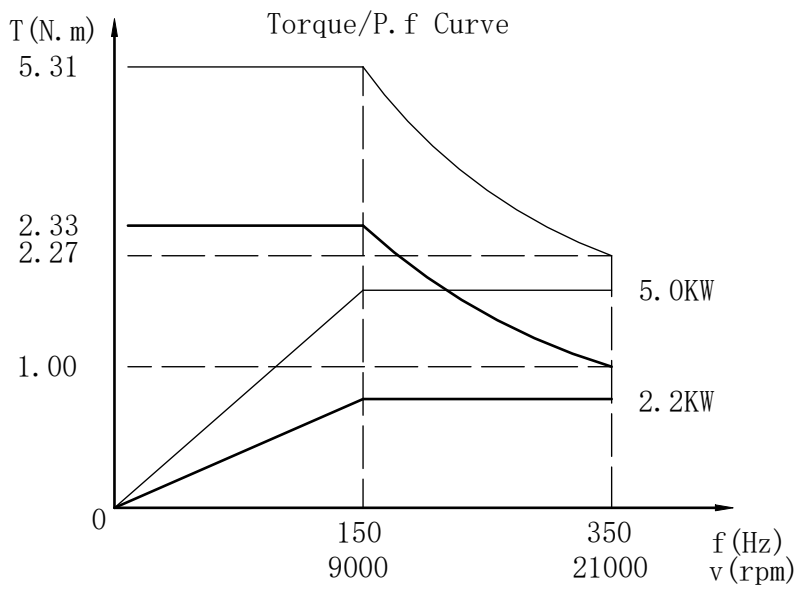
扭矩/功率曲线
